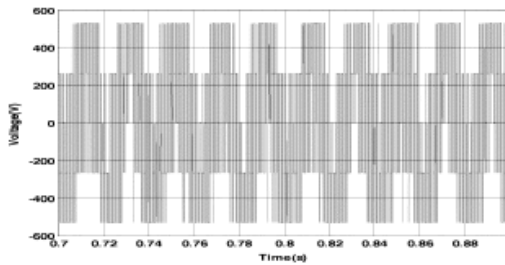
Fig. 8. STATCOM output voltage.
